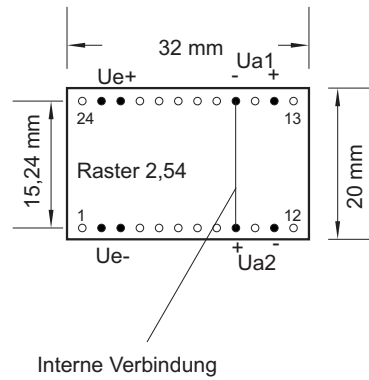
Anschlussplan: Durchsicht Duale Version
