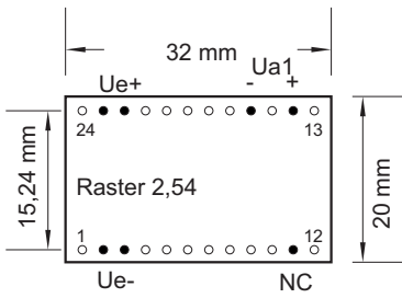
Anschlussplan: Durchsicht Single Version
